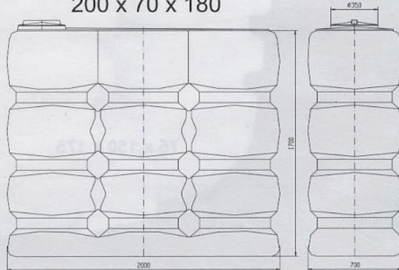
6594 REZERVOAR 2000 L 200 x 70 x 180
